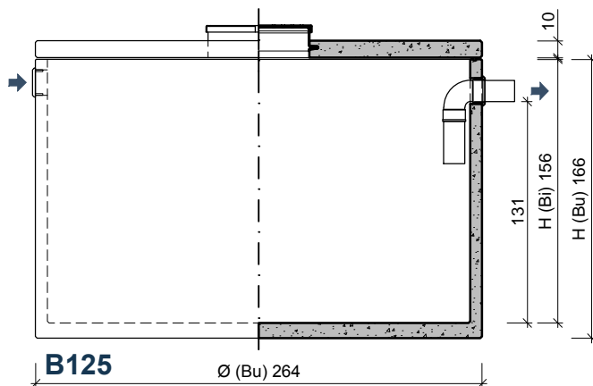
VOORAANZICHT / DOORSNEDE VUE FRONTALE / COUPE
