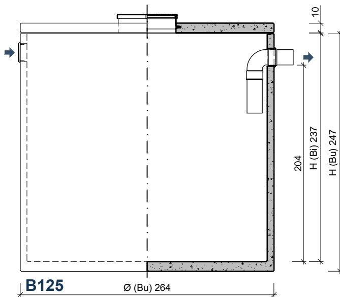
VOORAANZICHT / DOORSNEDE VUE FRONTALE / COUPE
